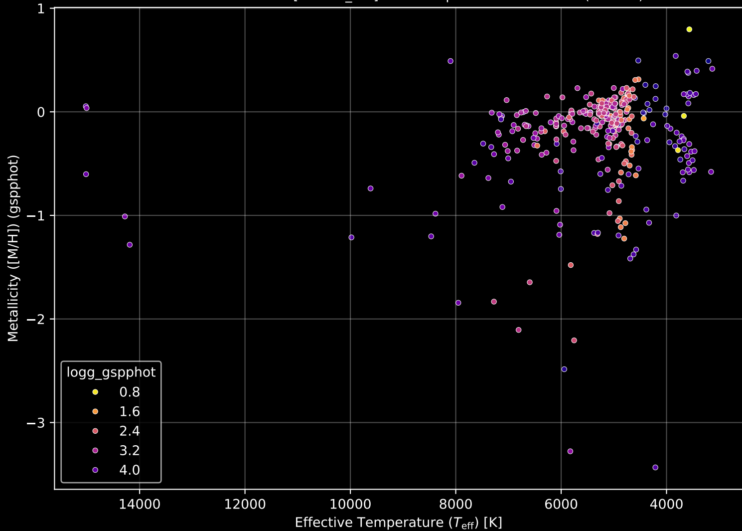
APOGEE DR17 Field: [160-18_btx] Stellar Population Parameters (n= 337)
